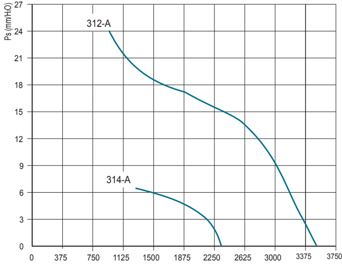
DUCT-M 310
