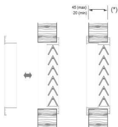
GPC Grilha de Passagem com Contra Aro
