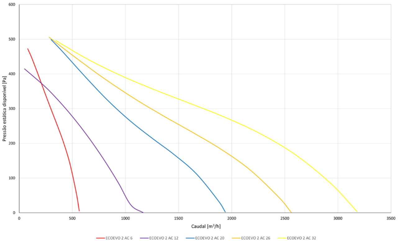
ECOEV0 2 AC e PM1 50% M5 + F7
